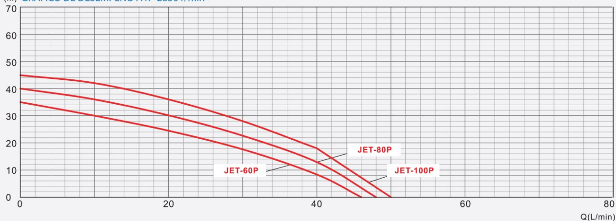
H (m) GRÁFICO DE DESEMPEÑO A n=2850 r/min
